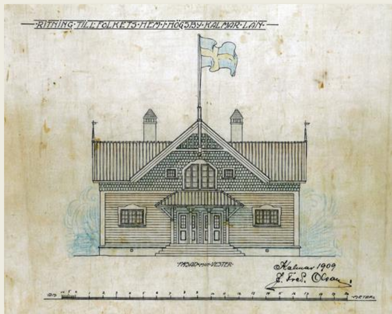
J. Fred. Olsons originalritning från 1909.
